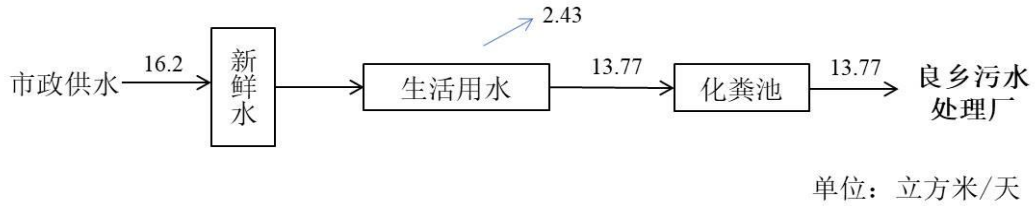
图3-6 日水平衡
