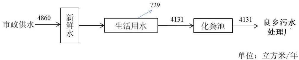
图3-7 年水平衡
